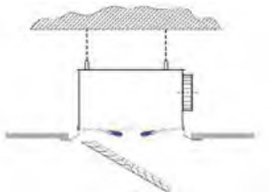
MONTAGGIO CON PLENUM FISSATO AL SOFFITTO
