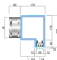
Dettaglio PSD altezza 50 mm con attacco S
