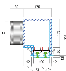
Dettaglio PS3F altezza 100 mm con attacco S
