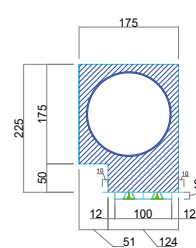
Dettaglio PS3F altezza 100 mm con attacco L
