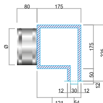
Dettaglio PSF altezza 30 mm con attacco S
