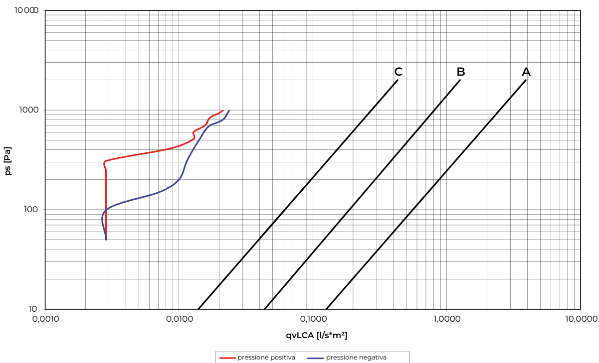
TENUTA ARIA TELAIO
