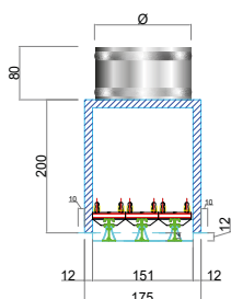
Dettaglio PS4F altezza 150 mm con attacco P
