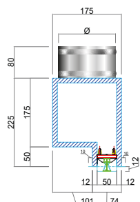
Dettaglio PS2F altezza 50 mm con attacco P
