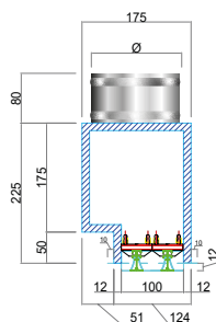
Dettaglio PS3F altezza 100 mm con attacco P
