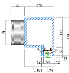
Dettaglio PS2F altezza 50 mm con attacco S
