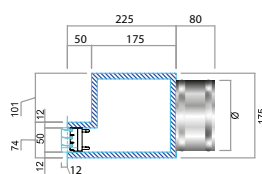
Dettaglio PSD altezza 50 mm con attacco P
