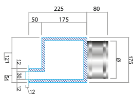
Dettaglio PSF altezza 30 mm con attacco P
