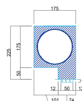
Dettaglio PSD altezza 50 mm con attacco L
